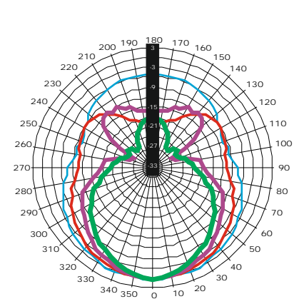
HORIZONTAL POLAR DIAGRAM — 250 — 500 — 1000 — 2000 — 4000 — 8000 — 12500 — 16000
