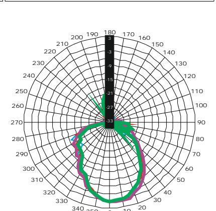
VERTICAL POLAR DIAGRAM — 9000 — 10000 — 12500 — 14000
