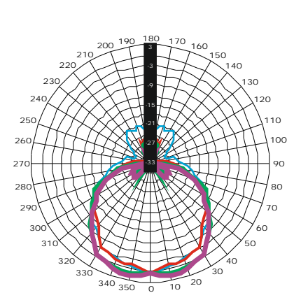
HORIZONTAL POLAR DIAGRAM — 250 — 500 — 1000 — 2000 — 4000 — 8000 — 12500 — 16000
