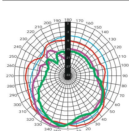
VERTICAL POLAR DIAGRAM — 250 — 500 — 1000 — 2000
